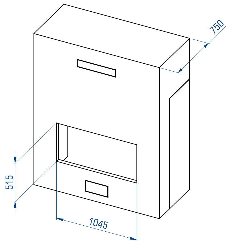
INSTALLAZIONE CON CORNICE FORNITA DALLA FABBRICA
