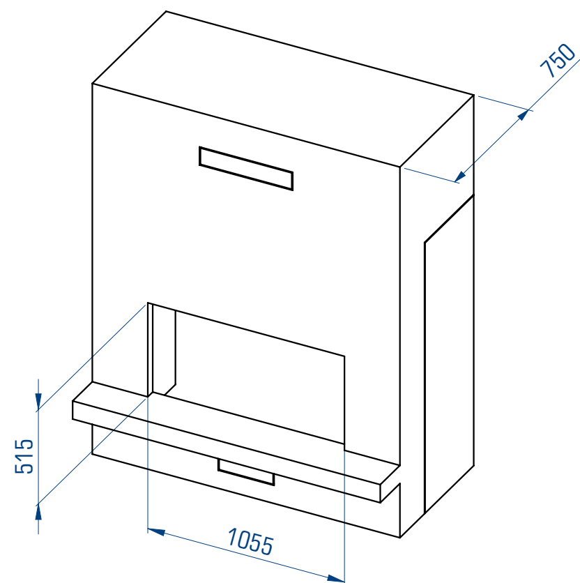
INSTALLAZIONE CON CORNICE 3 LATI KIT K0067AZ00
