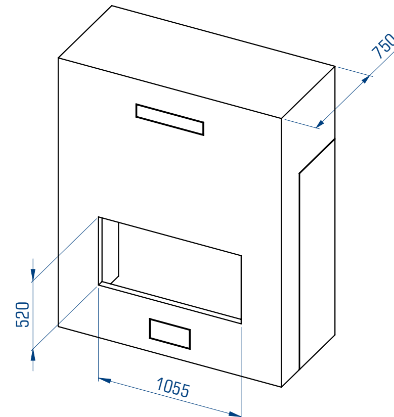
INSTALLAZIONE CON CORNICE 4 LATI KIT K0066AZ00
