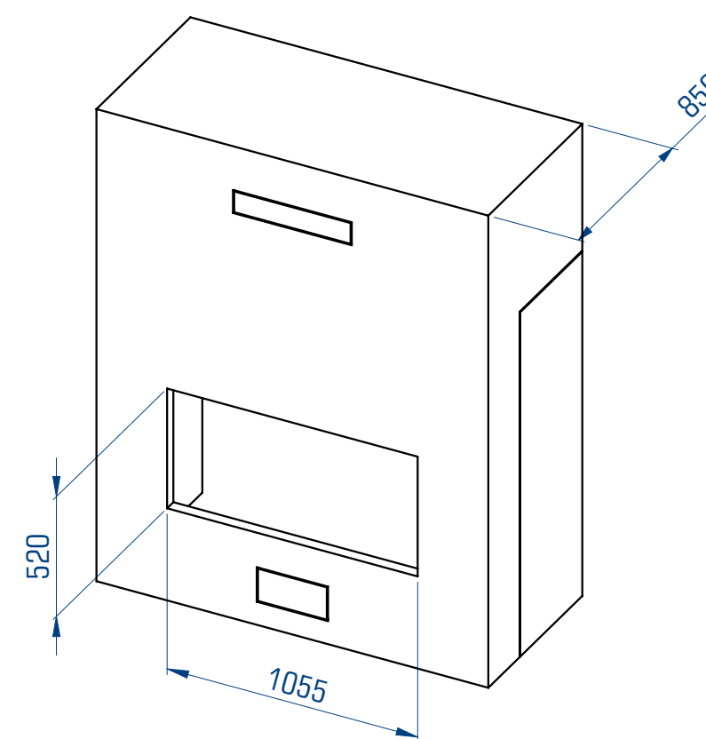
INSTALLAZIONE CON CORNICE INCASSATA KIT K0069AZ00
